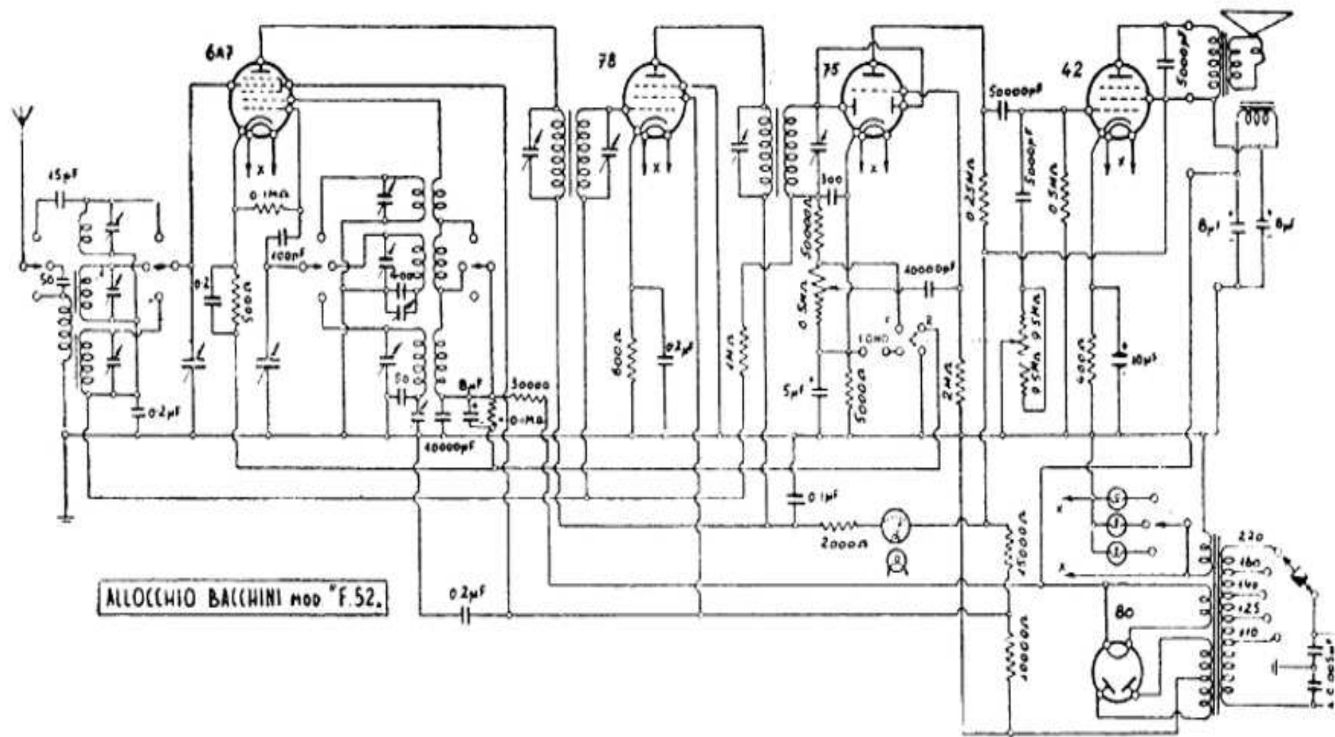
ALLOCCIO, BACCHINI e Co — Mod. F 52 M, Mod F 52 R e Mod F 52 G · Produzione 1937 Media frequenza 425 kHz.
